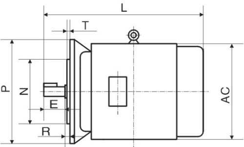
YE3-160~280
