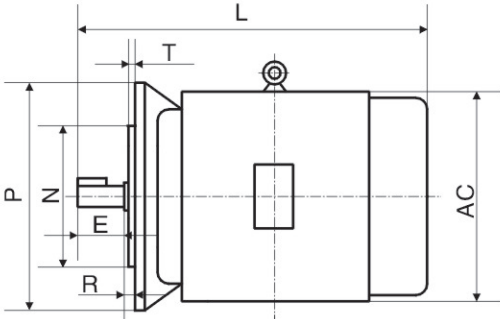
YE3-100~132
