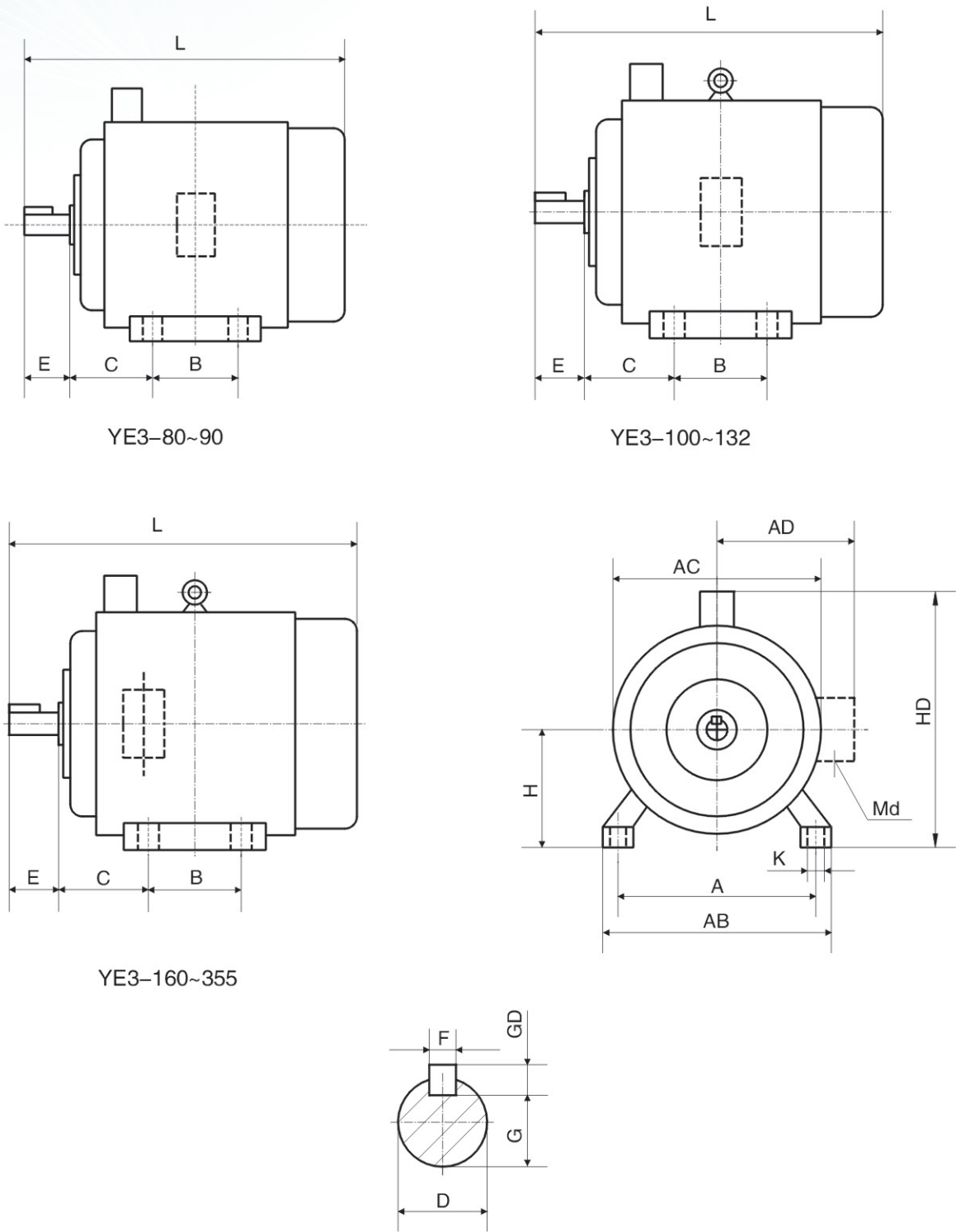
B3（机座号80~355）B6、B7、B8、V5、V6（机座号80~160）机座带底脚、端盖上无凸缘
