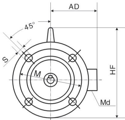
YE3-100~200
