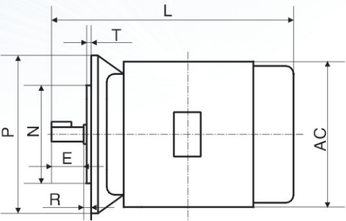
YE3-80~90
