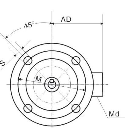
YE3-80~90
